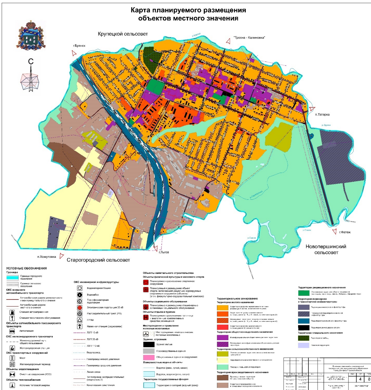
Рисунок – 1.4.9.1 - Карты (схемы) размещения водоснабжения МО город Дмитриев
